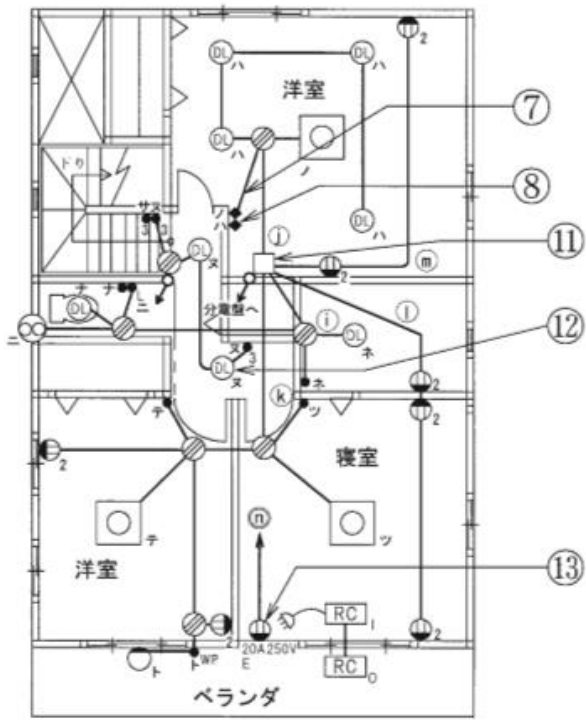
2階平面図
