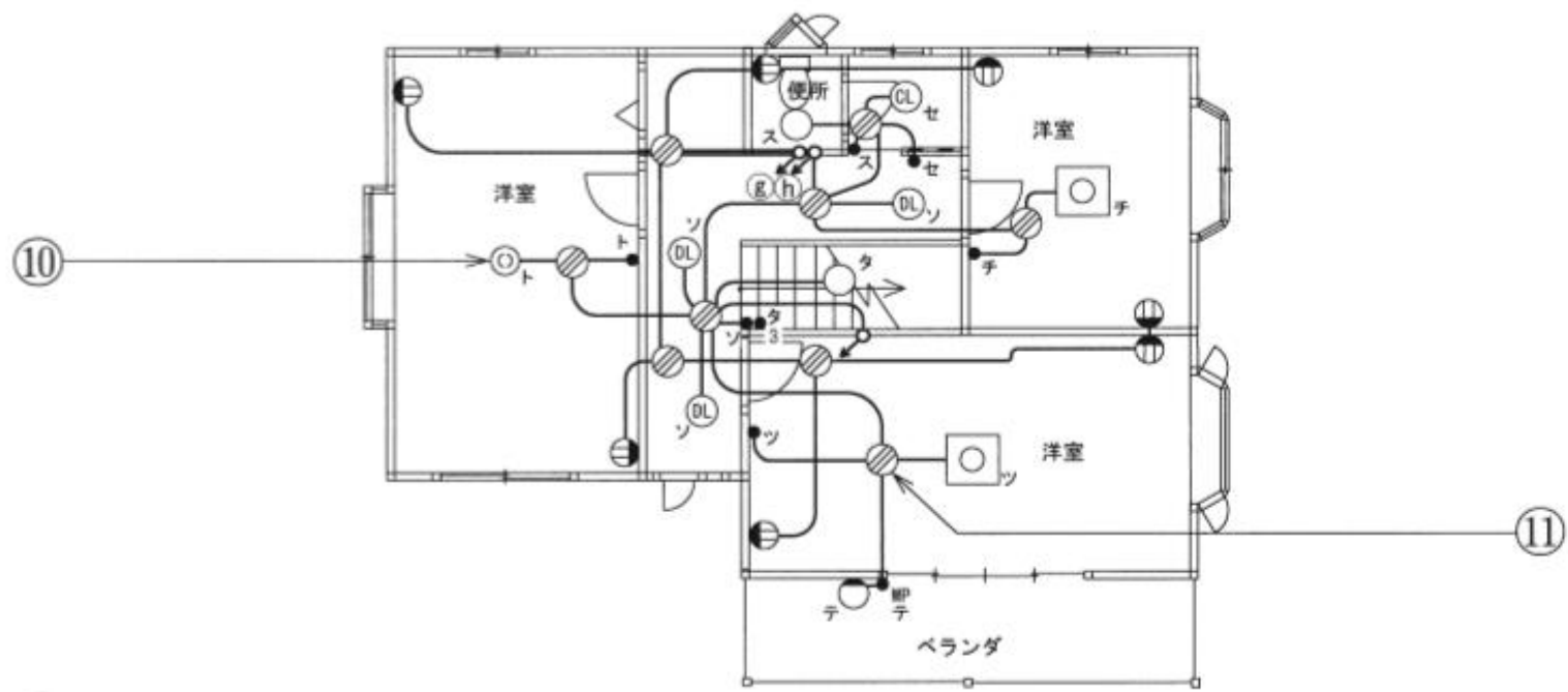
2階平面図
