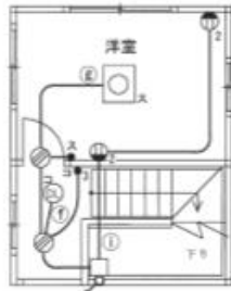
3階平面図
