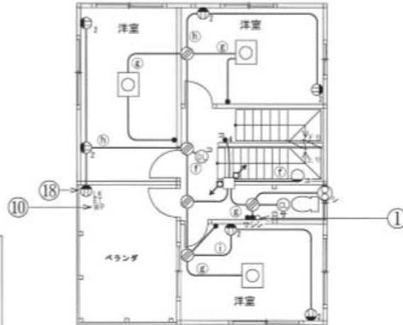
2階平面図
