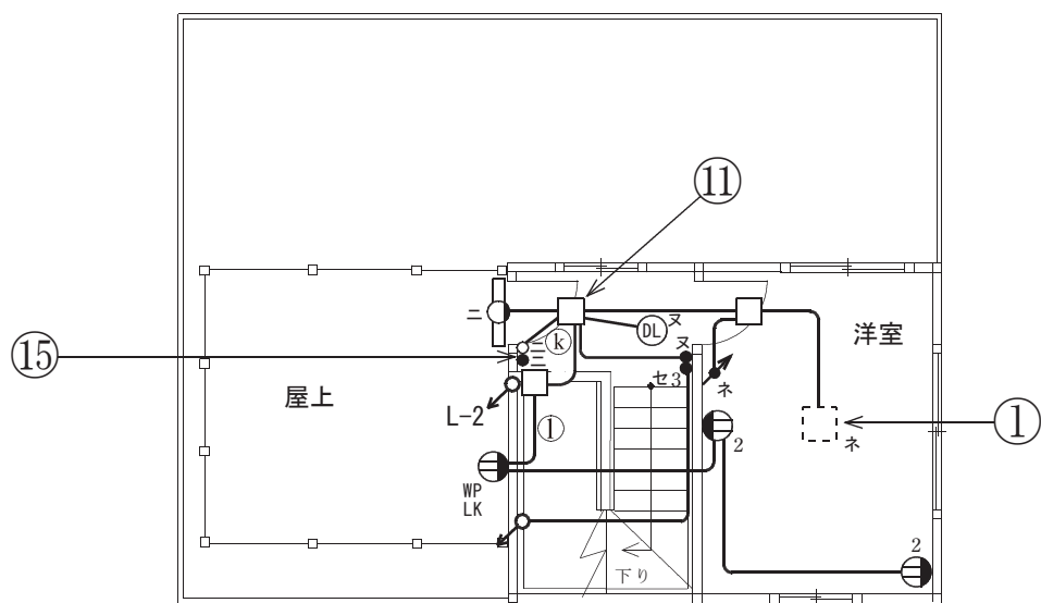
3階平面図
